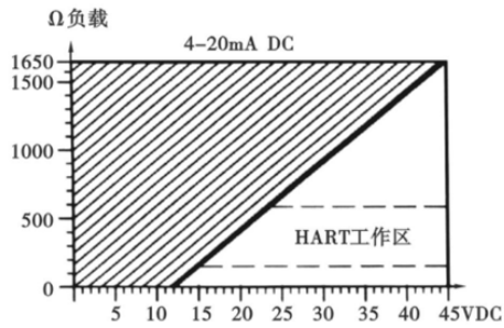
图2 负载特性图
